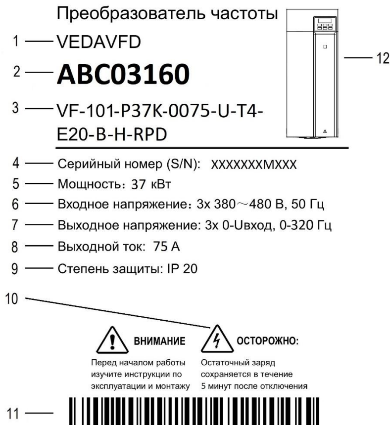
Рисунок 1.4-1. Пример маркировки преобразователя частоты VF-101 с прошивкой RPD
