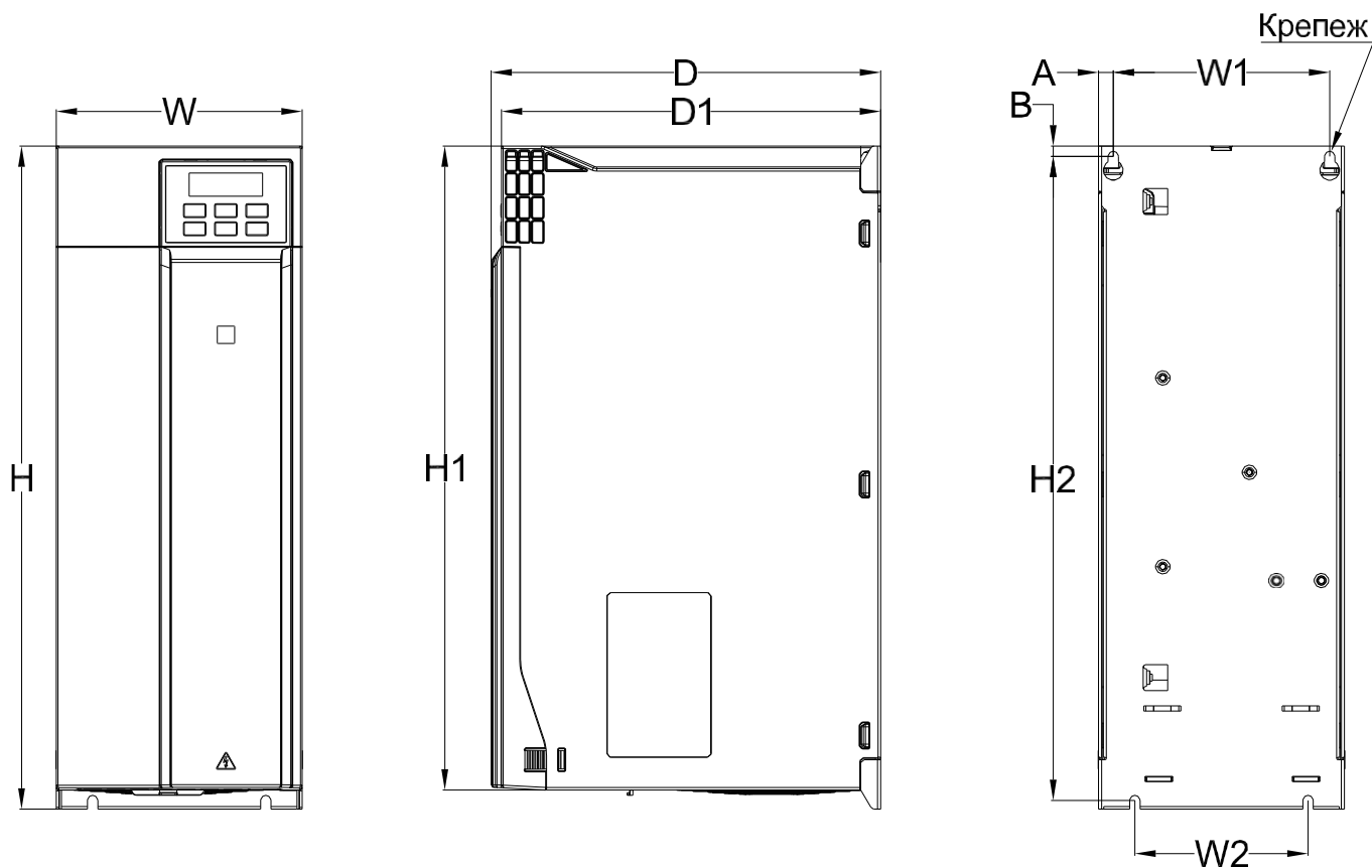
Рисунок 2.2-1 – Чертеж преобразователя частоты, типоразмер В4
