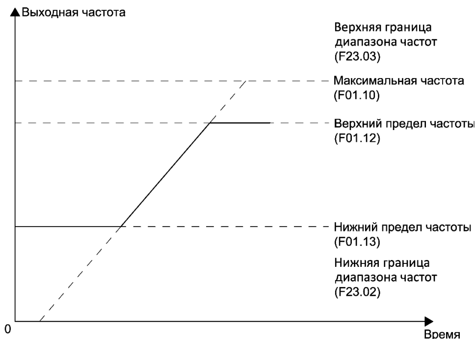
Рисунок 8.5-2 – Кривая выходной частоты, ограниченная верхним и нижним пределами В
