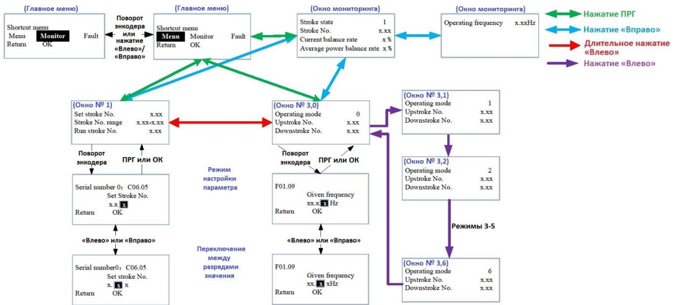
Рисунок 4.4-4 – Переключение между окнами графической панели управления при F23.13 = 2
