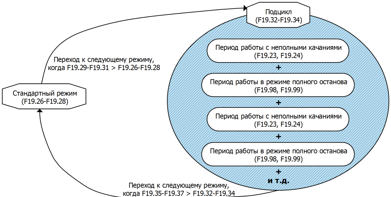
Рисунок 3.3-2 – Блок-схема циклического режима
