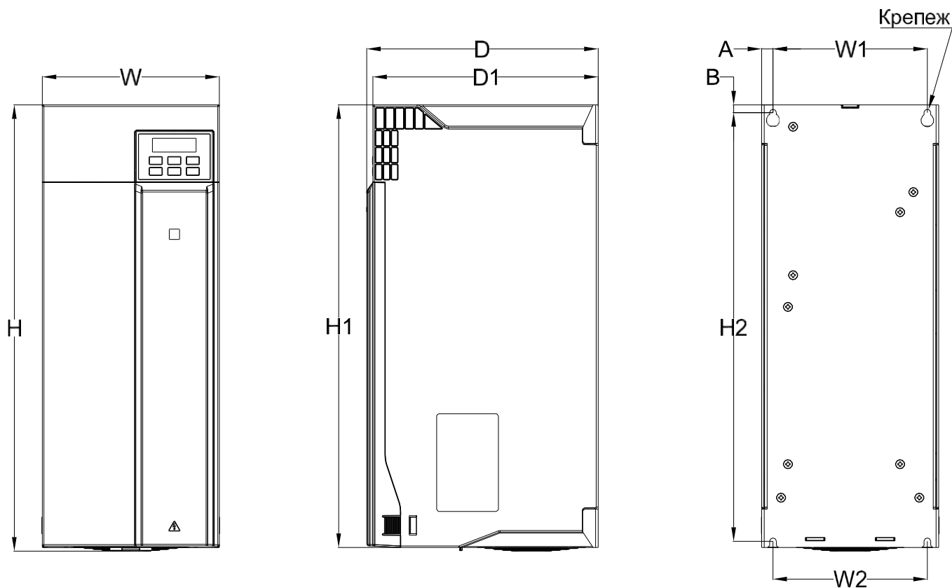
Рисунок 2.2-2 – Чертеж преобразователя частоты, типоразмер B5
