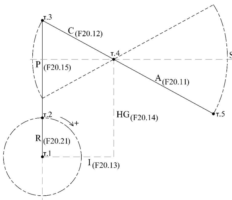
Рисунок 8.14-2 – Кинематическая схема станка-качалки
