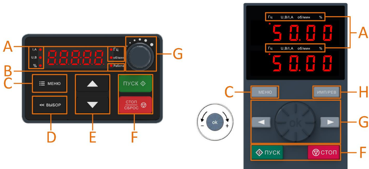
Рисунок 4.1-1 – Элементы панели управления преобразователя частоты
