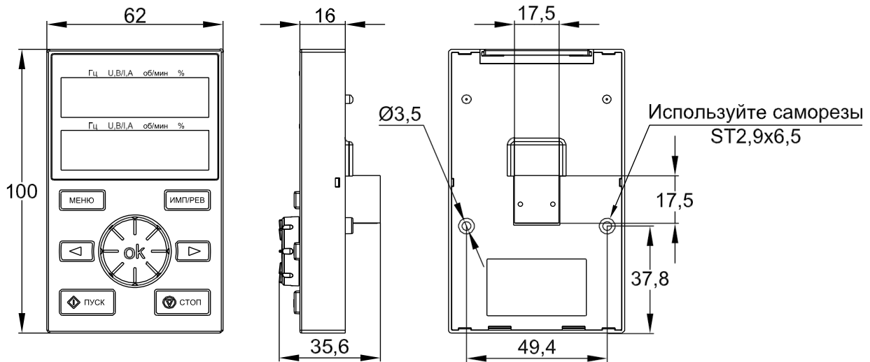
Рисунок 2.3-1 – Габаритные размеры и размеры отверстий внешней цифровой двухстрочной панели управления (единица измерения – мм)
