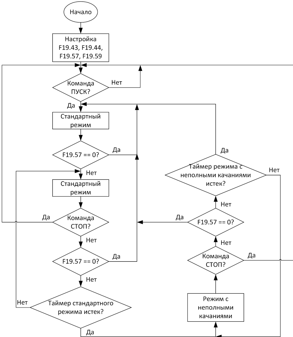
Рисунок 3.3-1 – Блок-схема прерывного режима с базовым чередованием (F19.59 = 0)
