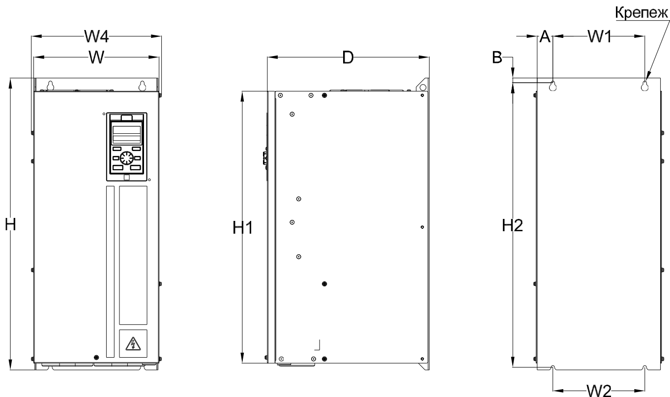
Рисунок 2.2-3 – Чертеж преобразователя частоты, типоразмер B6
