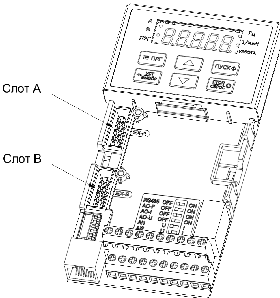
Рисунок 2.4-1 – Расположение слотов (разъемов) для установки опциональных карт на передней части преобразователя частоты
