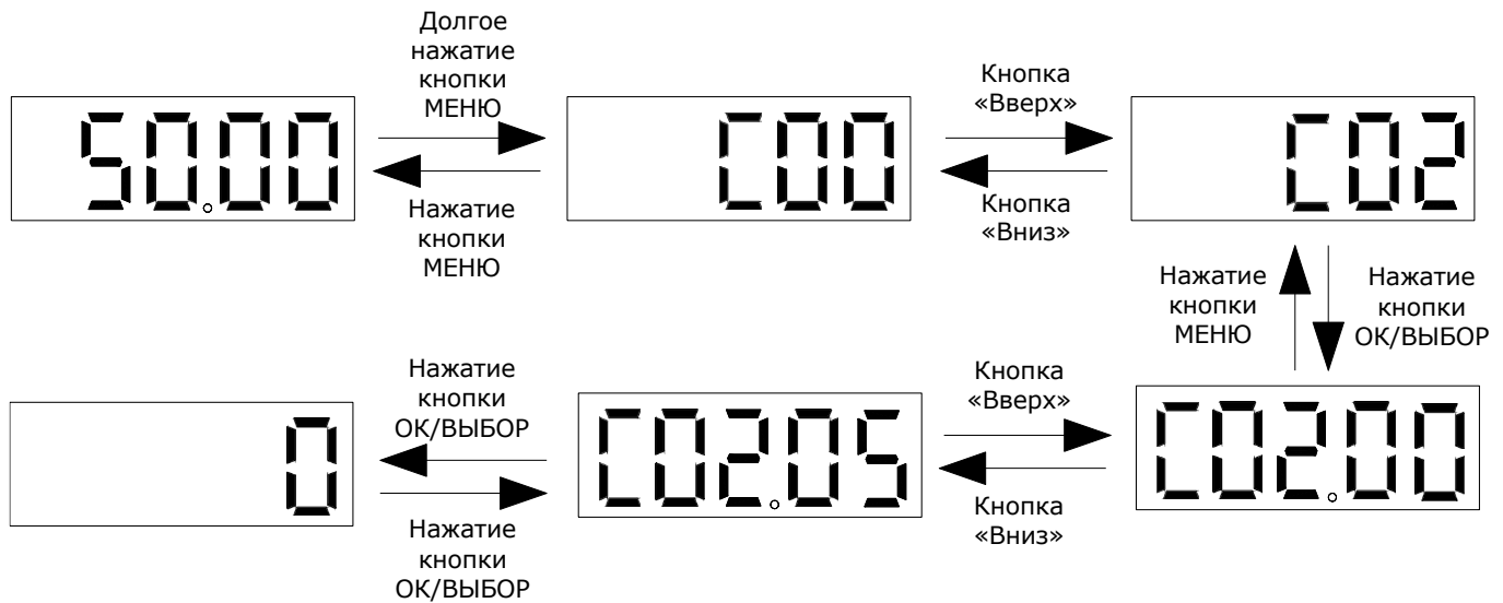
Рисунок 4.3-3 – Основные операции с панелью управления
