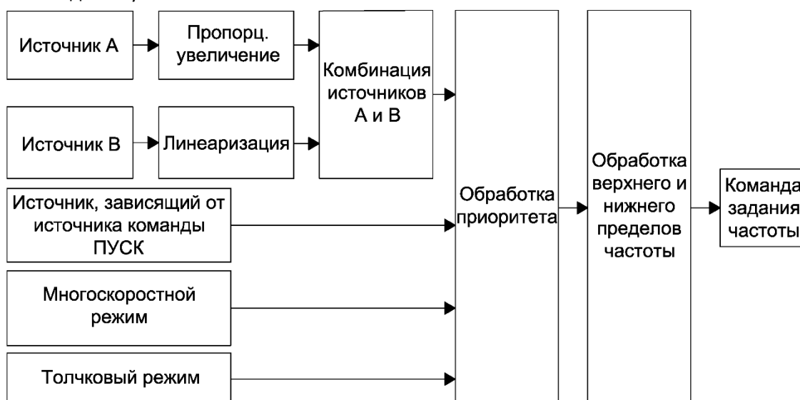
Рисунок 8.5-1 – Схема задания частоты
