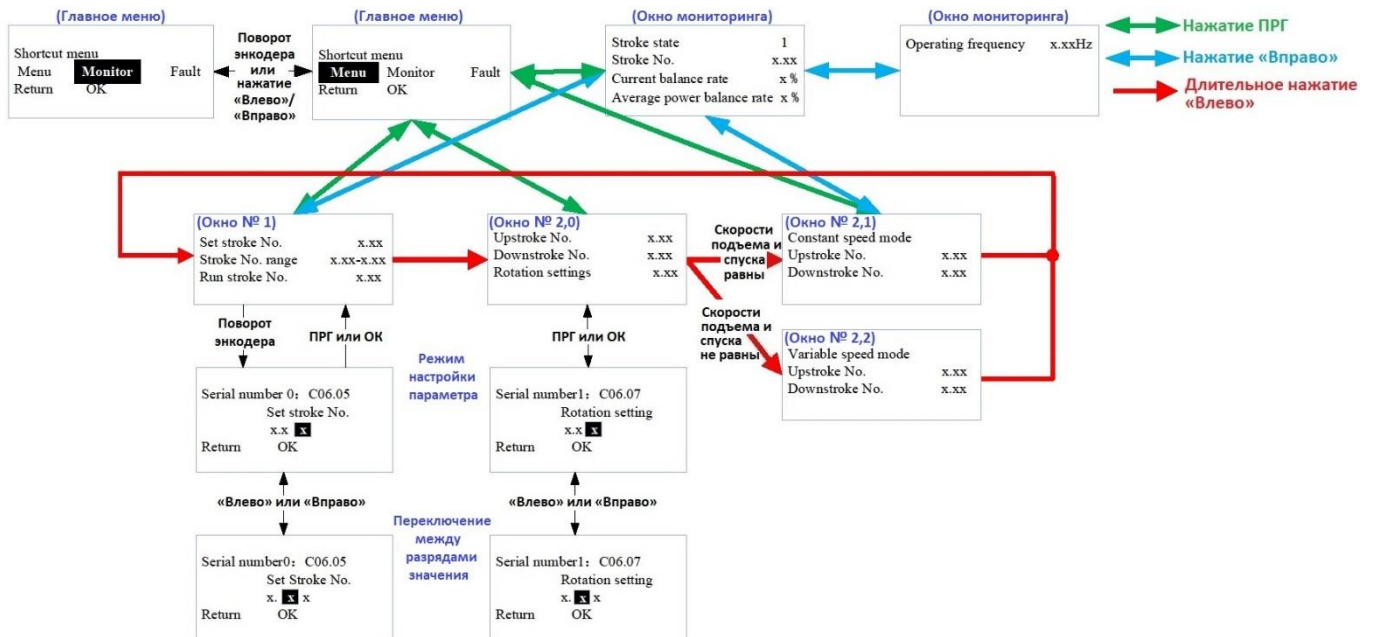
Рисунок 4.4-3 – Переключение между окнами графической панели управления при F23.13 = 1
