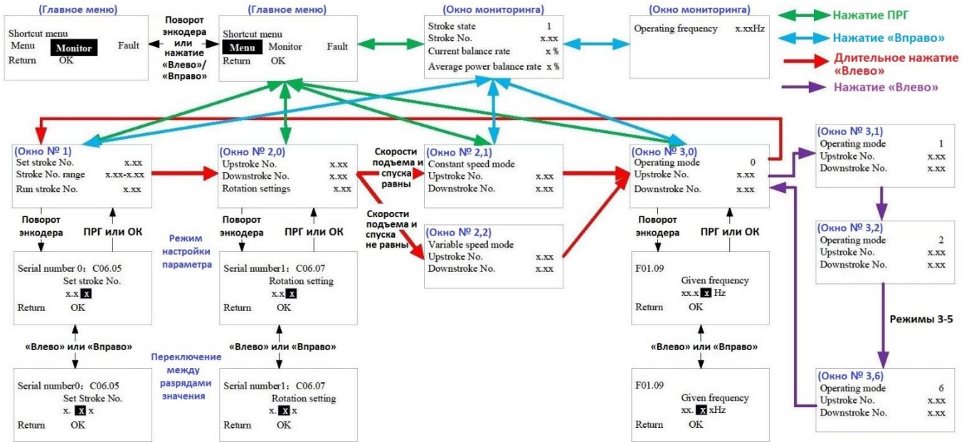
Рисунок 4.4-1 – Переключение между окнами графической панели управления при F23.13 = 3
