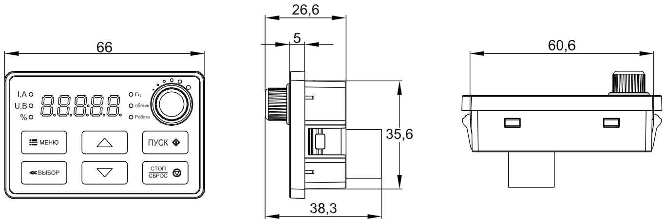
Рисунок 2.3-3 – Габаритные размеры и размеры отверстий внешней цифровой однострочной панели управления (единица измерения – мм)
