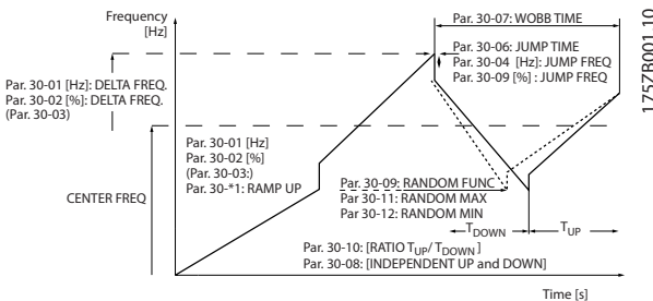
Рисунок 3.68 Генератор колебаний
