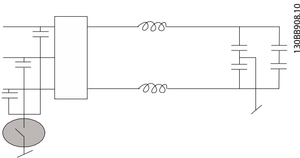
Рисунок 3.64 Фильтр ВЧ-помех
