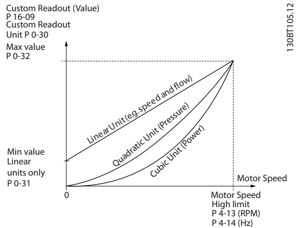
Рисунок 3.4 Показ.по выб.польз.
