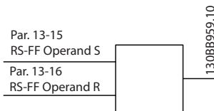
Рисунок 3.55 Триггеры сброса/установки
